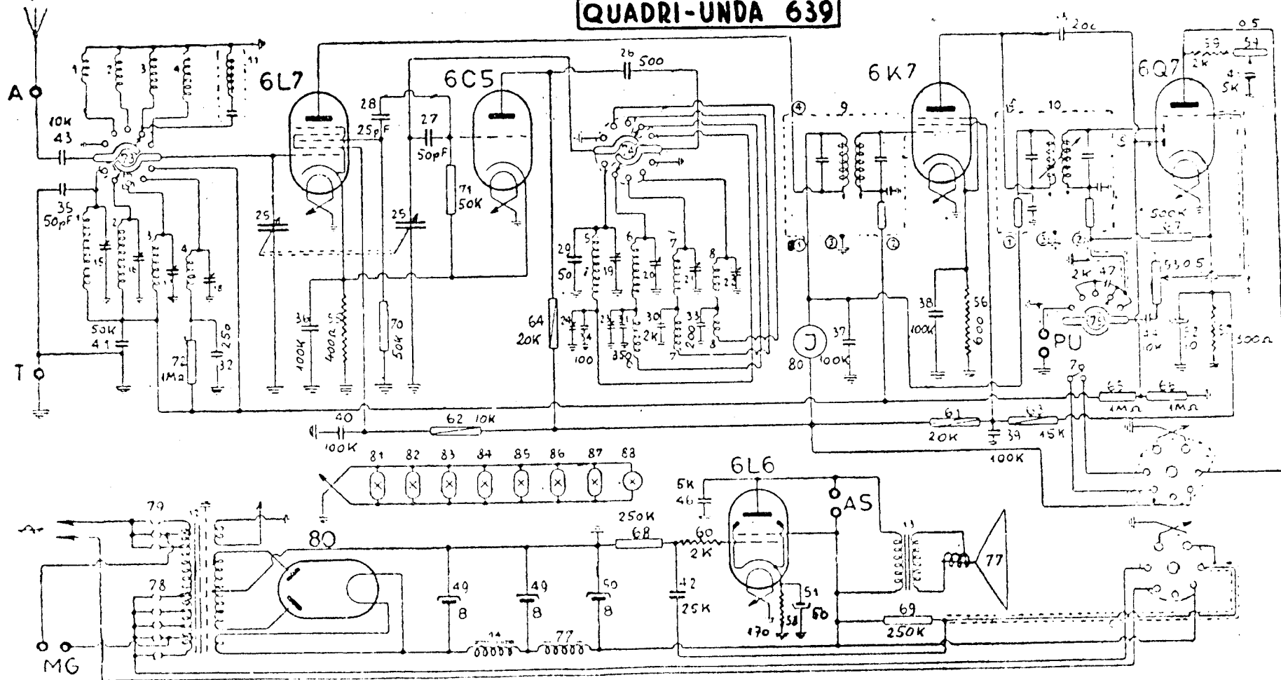
UNDA RADIO — Modello Super Quadri Unda 639. — Produzione 1938-39. — Gamme: cc. (15-30), c. (30-80), m. (206,5-600), l (870-1870) — Potenza d'uscita: 6,5 W — Media frequenza: 450 kHz
